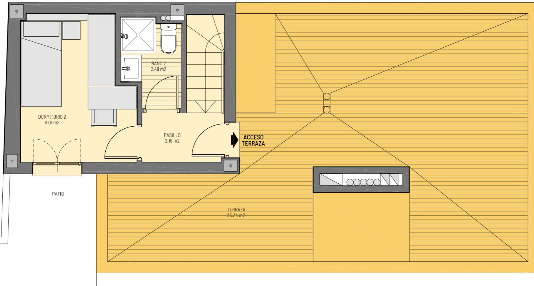
PLANTA ÁTICO
