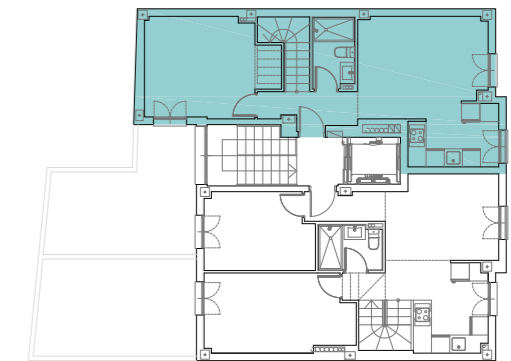
PLANTA SEGUNDA
